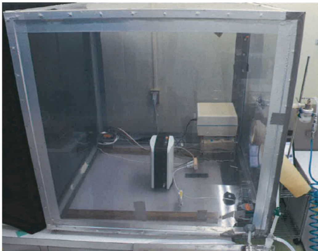
1m 3 試験チャンバー内の様子(中央に空気消臭除菌装置を設置)
